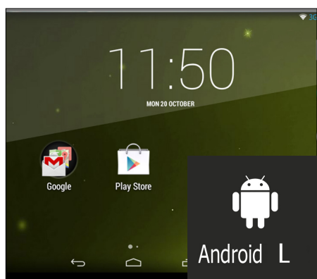
Android Lollipop 5.1
